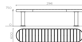
Tisch Best.-Nr. 16 170X
