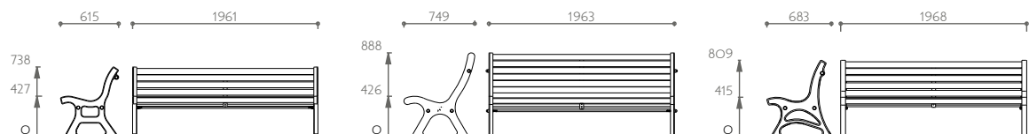
Royal 3-Sitzer Best.-Nr. 10 0050
