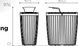
Easy mit Abfallsammlung von oben 2x 100 L Best.-Nr. 21 1210 S0E0 BOJL TR SW
