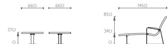
Niedriger Tisch Best.-Nr. 12 0240
