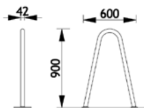
Umgekehrtes V Best.-Nr. 43 0171
