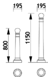
Poller aus Gusseisen Klassisch 3500 Best.-Nr. 40 351X NW
