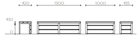
2-Sitzer-Bank ohne Rückenlehne Best.-Nr. 11 0502
