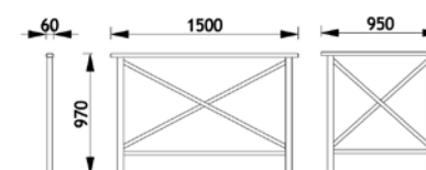
Modell 6600 Best.-Nr. 41 661X
