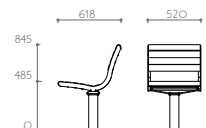
Solo Sitz Best.-Nr. 12 4510B
