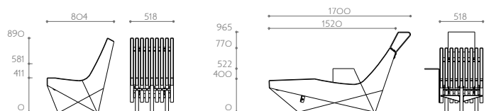
Liege Best.-Nr. 10 9150 mit Armlehne und Kopfstütze Best.-Nr. 10 9156
