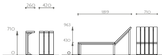
3 x Stehsitz Best.-Nr. 11 0504.P
