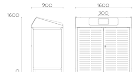
Sortierunterstand 660 L Best.-Nr. 61 0660
