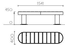
Kleine Sitzbank Best.-Nr. 16 160X
