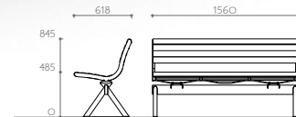
3-Sitzer-Bank Best.-Nr. 12 4530A
