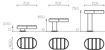
Niedriger Hocker Best.-Nr. 16 110X
