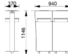
Diapason Duo 2x 75 L Mit Zigarettenlöscher Zum Einbetonieren: Best.-Nr. 27 0220 SOE0 0000 TR-TV Auf Grundplatte: Best.-Nr. 27 0221 SOE0 0000 TR-TV
