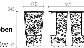
Easy grafisch 2x 110 L Best.-Nr. 20 1200 S0E0 00JL TR GRA
