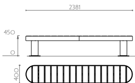
Bank Best.-Nr. 16 162X
