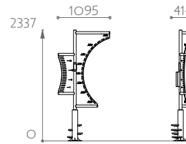
Senior-Bank 1 Benutzer 4 Übungen Best.-Nr. 07 109
