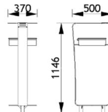
Diapason 75 L Mit Zigarettenlöscher Zum Einbetonieren: Best.-Nr. 27 0200 Auf Grundplatte: Best.-Nr. 27 0201
