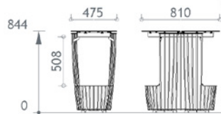
Easy mit frontaler Abfallsammlung 2x 100 L Best.-Nr. 21 1200 S000 00J0 TR
