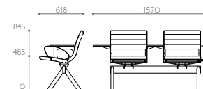
Duo nebeneinander mit 2 Ablagen und 1 Armlehne Best.-Nr. 12 4521A-01
