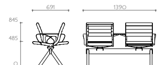
Duo Sitz Face to Face mit 1 Ablage und 2 Armlehnen Best.-Nr. 12 4521A-02
