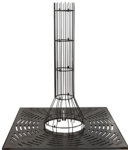
Baumschutzgitter 5000 Best.-Nr. 42 5000
