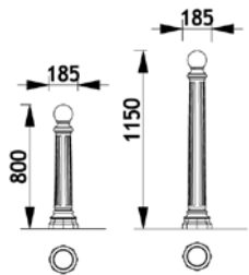
Poller aus Gusseisen Style 3400 Best.-Nr. 40 341X NW
