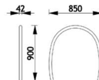
Bogen breit Best.-Nr. 43 0151
