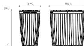
Easy mit Abfallsammlung von oben 1x 100 L | 2x 50 L Best.-Nr. 21 1230 S0E0 BOJL TR
