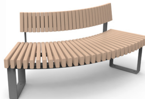
Gebogen 3-Sitzer-Bank Innendurchmesser Ø 2,12 m Außendurchmesser Ø 3,06 m Best.-Nr. 10 3436
