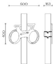
Einfache Silhouette Best.-Nr. 43 50X1
