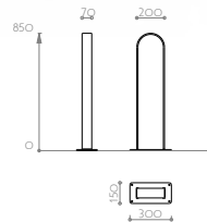
U flach schmal Best.-Nr. 43 4001
