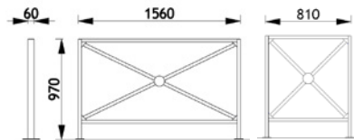
Modell 6000 Best.-Nr. 41 601X
