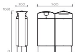
Eidos 1x 12 L + 1x 44 L | 1x 56 L Best.-Nr. 20 0420 B2C1 0F00 TR-TV VG3
